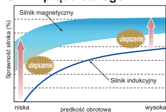
Silnik prądu stałego
